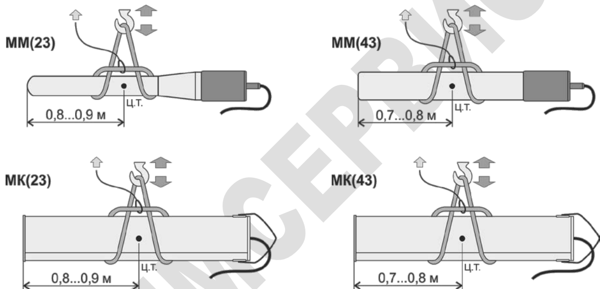
Рисунок 2 – Схема строповки заземлителей конструктивного исполнения ММ и МК при укладке в траншею
