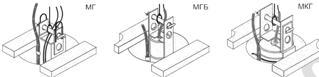
Рисунок 10 – Схема строповки гирлянды заземлителей
