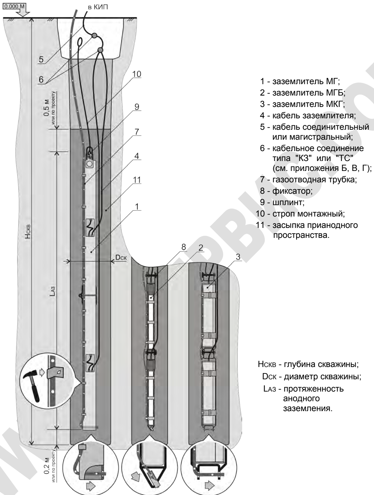
Рисунок 5 – Схема глубинного анодного заземления на базе анодных заземлителей МГ, МГБ, МКГ
