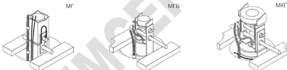
Рисунок 9 – Схема стыковки заземлителей в устье скважины
