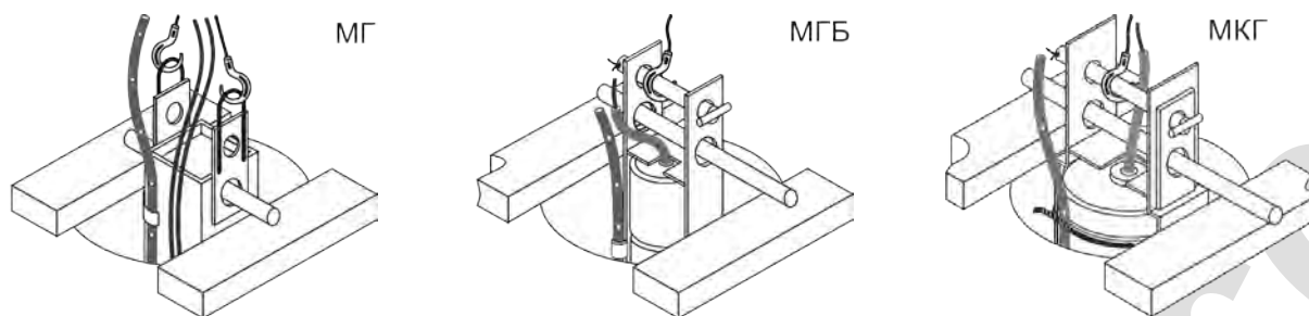
Рисунок 8 – Схема фиксирования заземлителя в устье скважины
