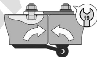
Рисунок 7 – Схема соединения секций
