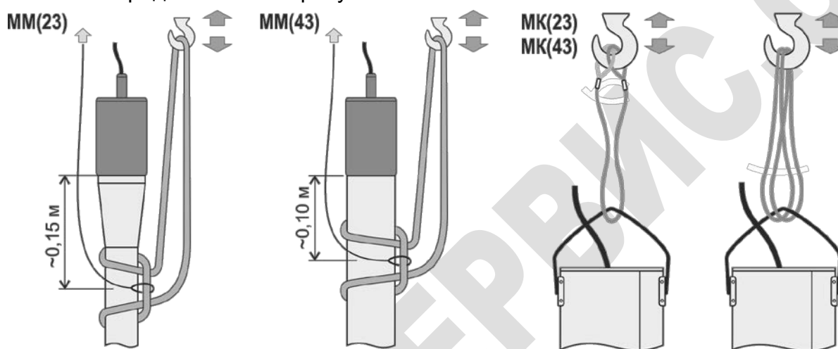
Рисунок 4 – Схема строповки заземлителей ММ и МК при установке в скважину
